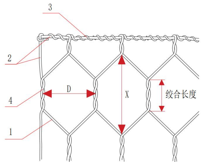
图 2 生态格网示意图
