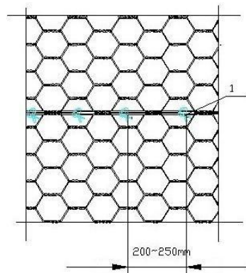
图 10.3.1-3 扎丝绑扎示意图
