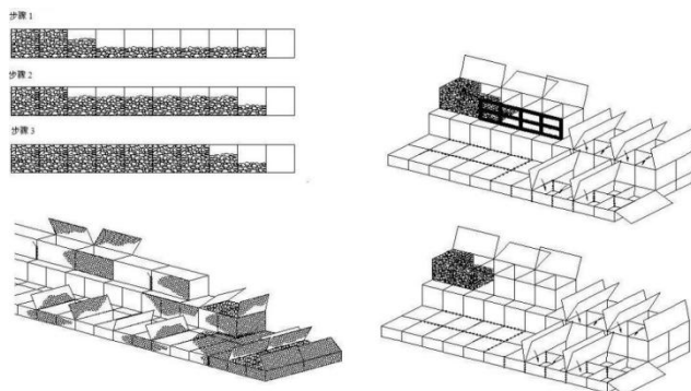
图 10.4.1 固滨笼组合体填石示意图
