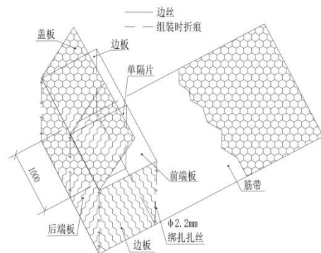
图7.2.1-2 加筋固滨笼示意图
