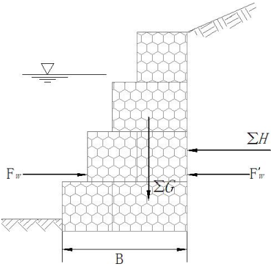
图 8.3.1 固滨笼挡土墙受力简图
