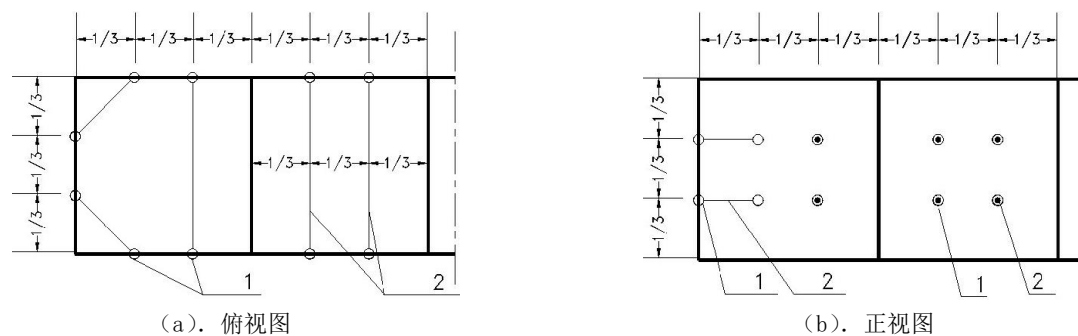
图 10.4.4 固滨笼内部连接加强钢丝绑扎示意
