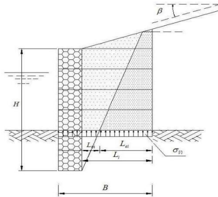
图 8.5.3 加筋固滨挡墙内部稳定计算简图
