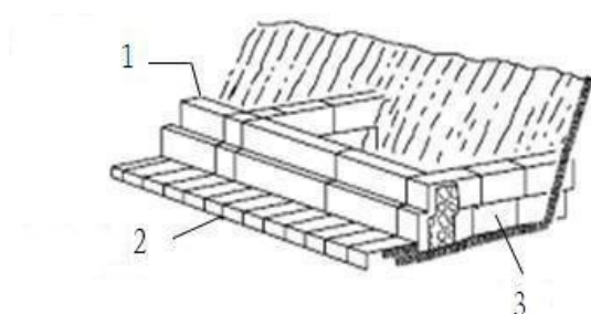
图 3 带扶壁的河道整治挡墙
